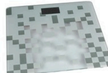
15K10607 客房电子秤 Rooms electronic scales 尺寸/Size: 300x320x21mm 最大秤量 /Maximum capacity: 150Kg
